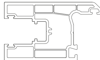
OUVRANT COULISSANT
